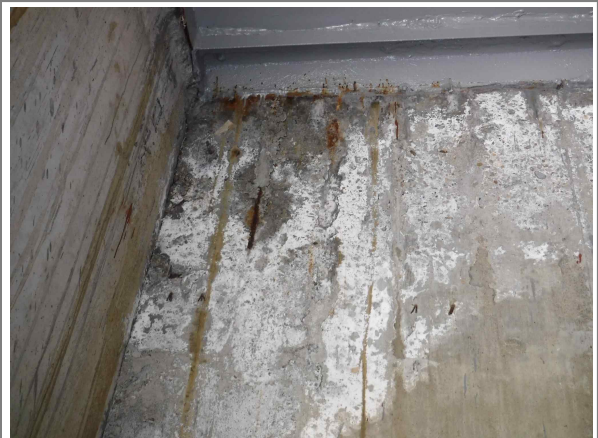
도면번호 : 70 바닥판 가로보 S15 손상현황 : 03 백태/박리/철근노출
