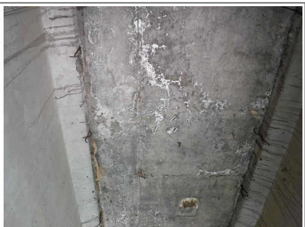
도면번호 : 24 바닥판 하면 S5 손상현황 : 03 망상균열/백태
