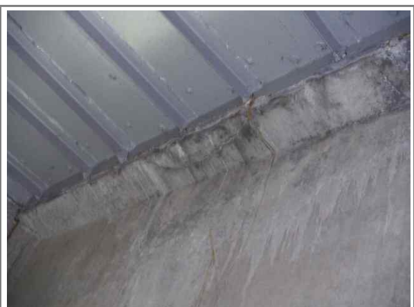
도면번호 : 50 PSCI 거더 S13 G1 손상현황 : 05 균열
