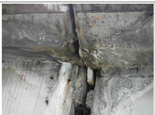
도면번호 : 22 바닥판 하면 S3 손상현황 : 05 조인트파손
