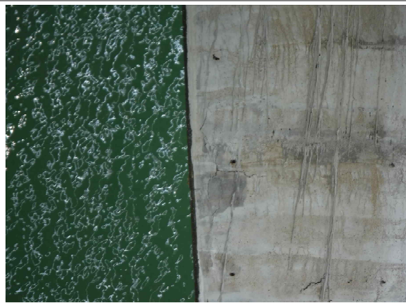
도면번호 : 84 교각 P9 손상현황 : 07 박리
