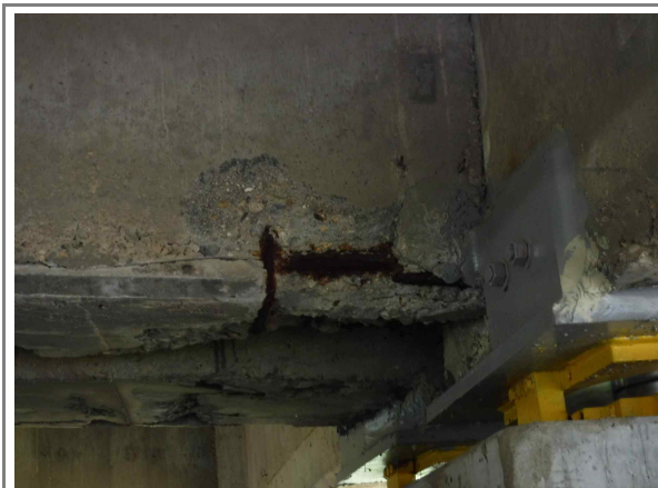
도면번호 : 70 바닥판 가로보 S15 손상현황 : 13 박락/철근노출
