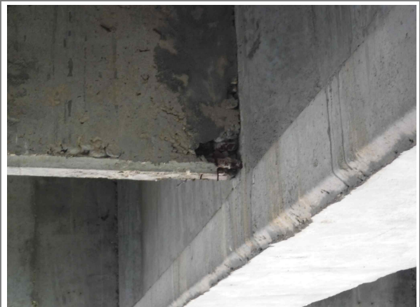
도면번호 : 65 바닥판 가로보 S10 손상현황 : 07 재료분리/철근노출
