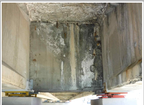
도면번호 : 68 바닥판 가로보 S13 손상현황 : 01 백태
