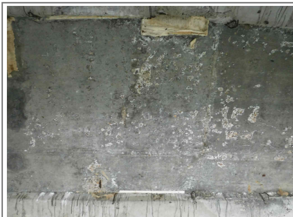
도면번호 : 24 바닥판 하면 S5 손상현황 : 02 망상균열/백태
